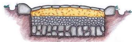
Struktura cestišča
